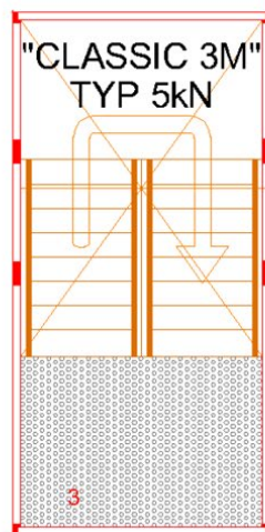
1. OBERGESCHOSS
